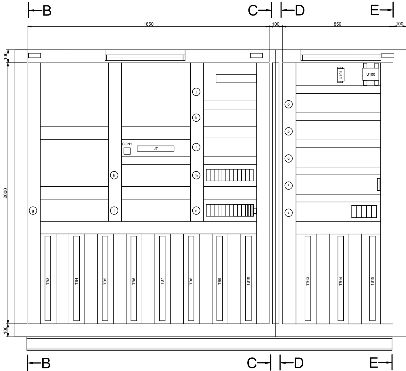
Вид спереди без дверей
